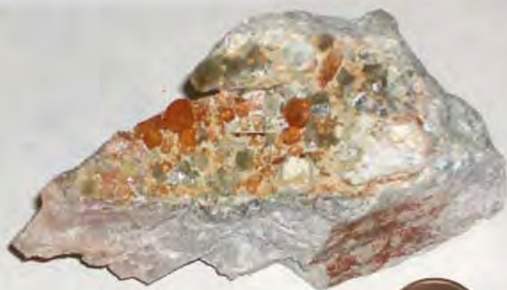
▲ Хромистый гроссуляр в родингите ▼ Гроссуляр и диопсид на родингите
